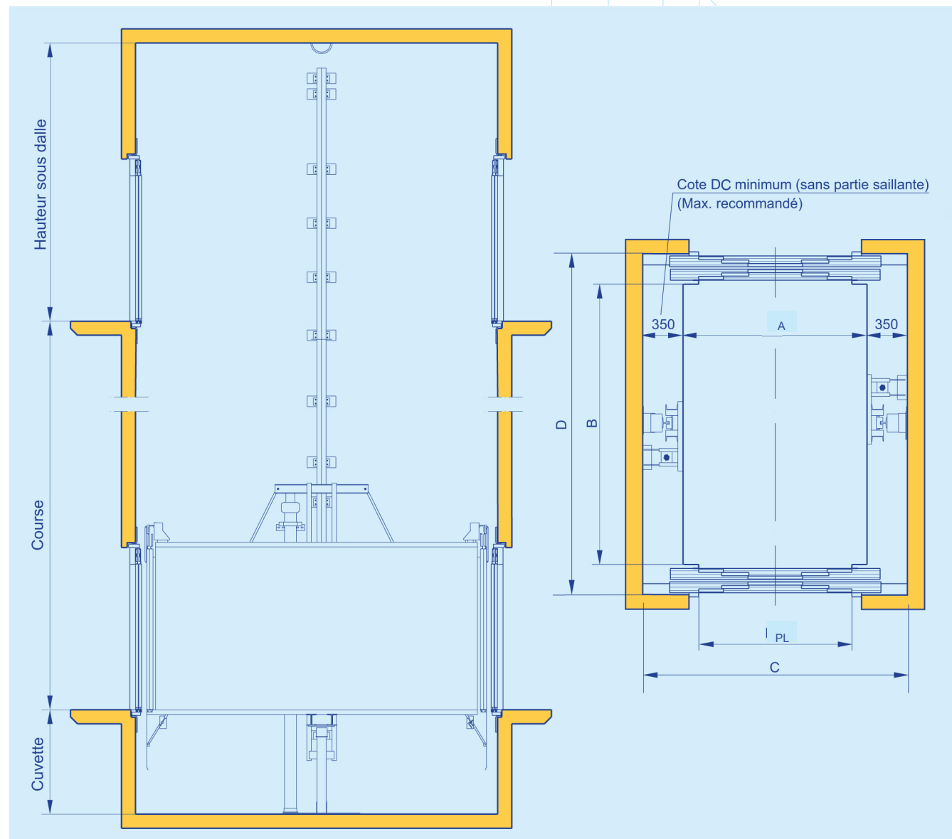
Figure 5: Ce modèle est un ascenseur hydraulique à action directe, qui n'est valable que pour l'ordre de courses décrit ci-dessous. Dans l'ordre de course spécifié, nous fournissons ce modèle et non le modèle MIH (hydraulique à action directe). Il est plus simple que le MIH, car il est dépourvu de chaînes de tractions, de boîtiers de poulies, de limiteurs de vitesse et de guide de vérin. Les portes livrées sont de la marque Wittur.
