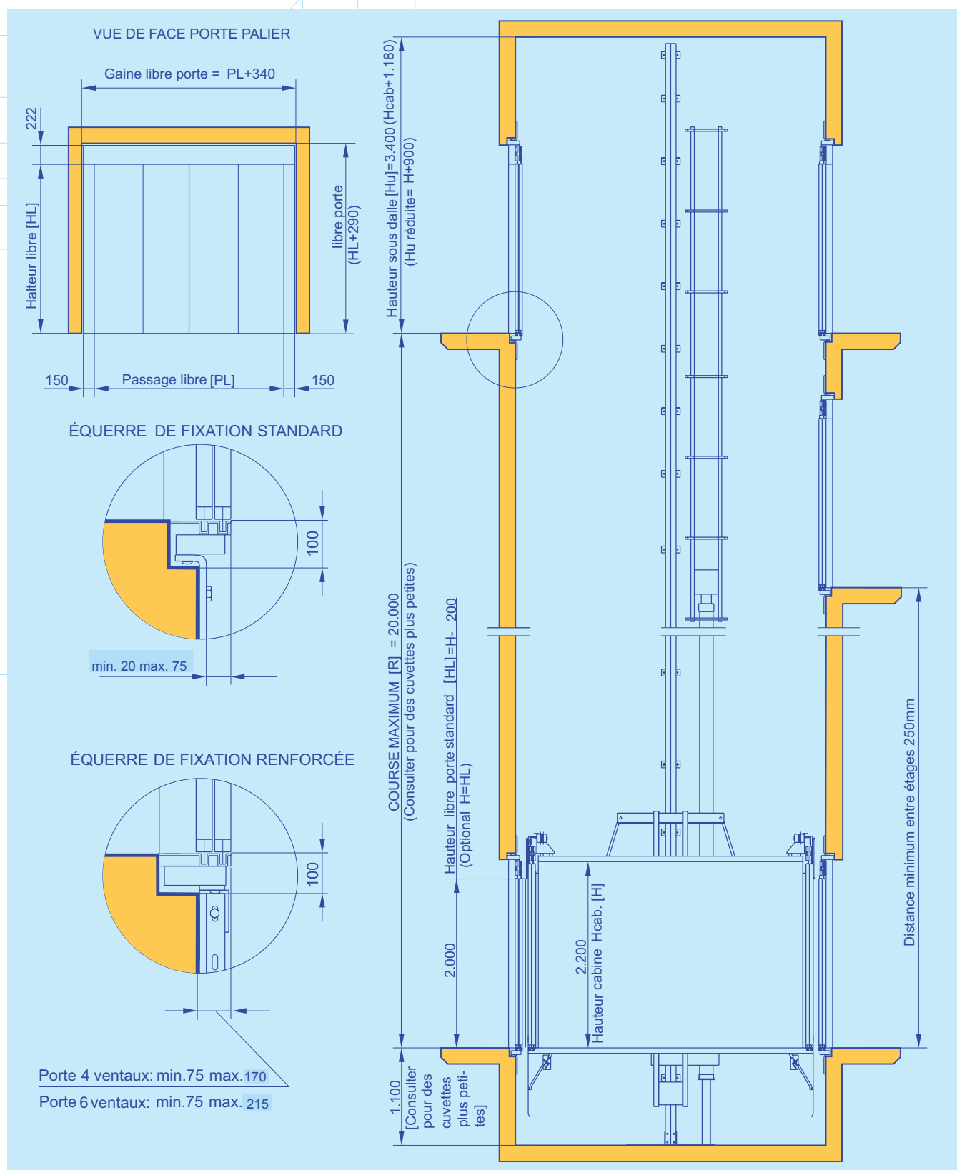
Figure 6: Voici un exemple de mesure standard, avec Hauteur Cabine = 2.200mm. Les portes fournies sont de la marque Wittur.
