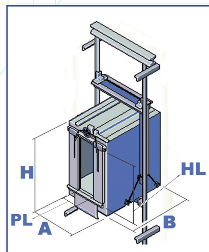
Figure 4: Schéma de dimensions de carlingue.
