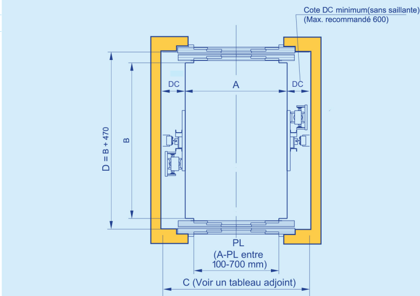
Figure 8: Dimensions minimales de gaine (étage). Opérateur automatique central à 6 vantaux en cabine. Portes automatiques à 6 vantaux à ouverture centrale.
