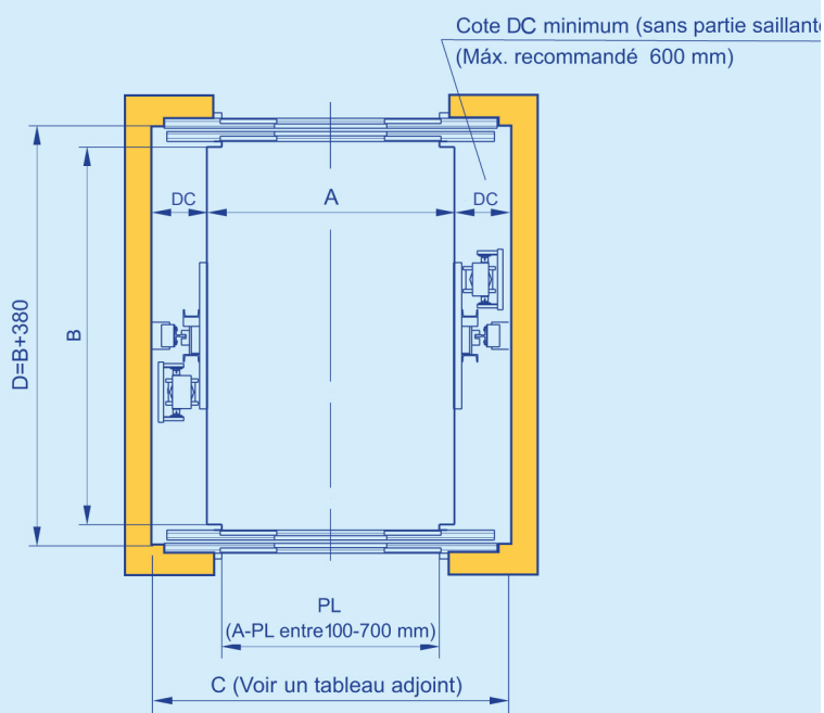
Figure 7: Dimensions minimales de gaine (étage). Opérateur automatique central à 4 vantaux en cabine. Portes automatiques à 4 vantaux à ouverture centrale sur paliers.
